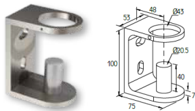
ΕΞΩΤΕΡΙΚΟ ΣΤΗΡΙΓΜΑ ΚΟΛΩΝΑΣ F50-100/103 EXTERNAL SUPPORT FOR F50-100/103 COLUMN Κωδ. / Code 4143
