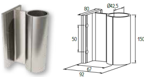
ΕΞΩΤΕΡΙΚΟ ΕΠΙΤΟΙΧΙΟ ΣΤΗΡΙΓΜΑ ΓΙΑ ΚΟΛΩΝΑ Ø42 EXTERNAL WALL SUPPORT FOR COLUMN Ø42 Κωδ. / Code 4194
