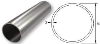
ΚΟΥΠΙΑΣΤΗ Ø50 HANDRAIL Ø50 Κωδ. / Code F50-200
