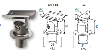
ΣΥΝΔΕΣΜΟΣ ΚΟΥΡΙΑΣΤΗΣ Ø50 ΜΕ ΚΟΛΩΝΑ Ø42 (ΣΚΑΛΑ) CONNECTOR FOR HANDRAIL Ø50 WITH COLUMN Ø42 (STAIRS)
