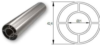
ΚΟΛΩΝΑ ΣΤΗΡΙΞΗΣ Ø42 SUPPORT COLUMN Ø42 Κωδ. / Code F50-100
