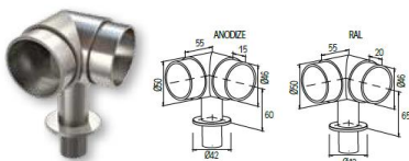
ΣΥΝΔΕΣΜΟΣ 90° ΓΙΑ ΚΟΥΡΙΑΣΤΗ Ø50 CONNECTOR 90° FOR HANDRAIL Ø50
