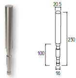
ΕΝΔΟΔΑΠΕΔΙΟ ΣΤΗΡΙΓΜΑ ΓΙΑ ΚΟΛΩΝΑ Ø42 INFLOOR SUPPORT FOR Ø42 COLUMN
