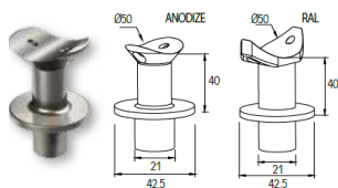
ΣΥΝΔΕΣΜΟΣ ΚΟΥΡΙΑΣΤΗΣ Ø50 ΜΕ ΚΟΛΩΝΑ Ø42 CONNECTOR FOR HANDRAIL Ø50 WITH COLUMN Ø42
